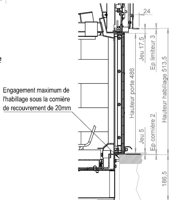
Coupe transversale A-A (1 : 8)
